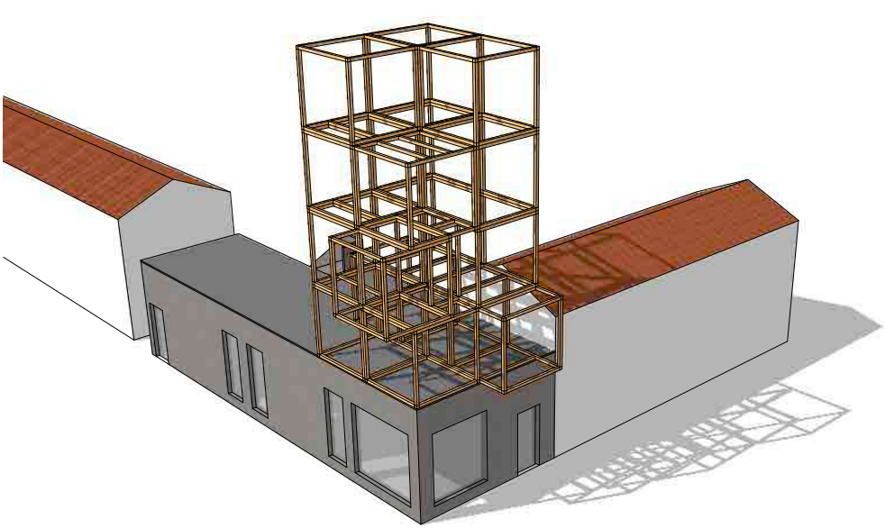
CONSTRUCTIE houten skelet
